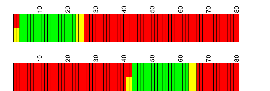
VREMENSKI PLAN RADA SEMAFORSKIH UREĐAJA (SIGNALNI PLAN)
