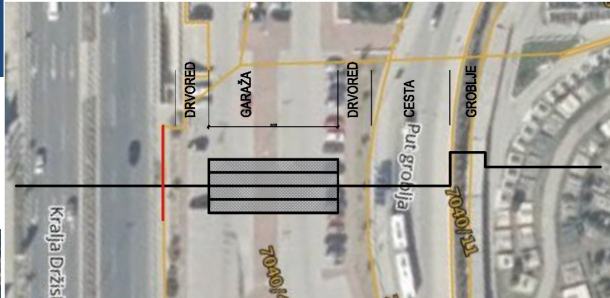
Shematski presjek
